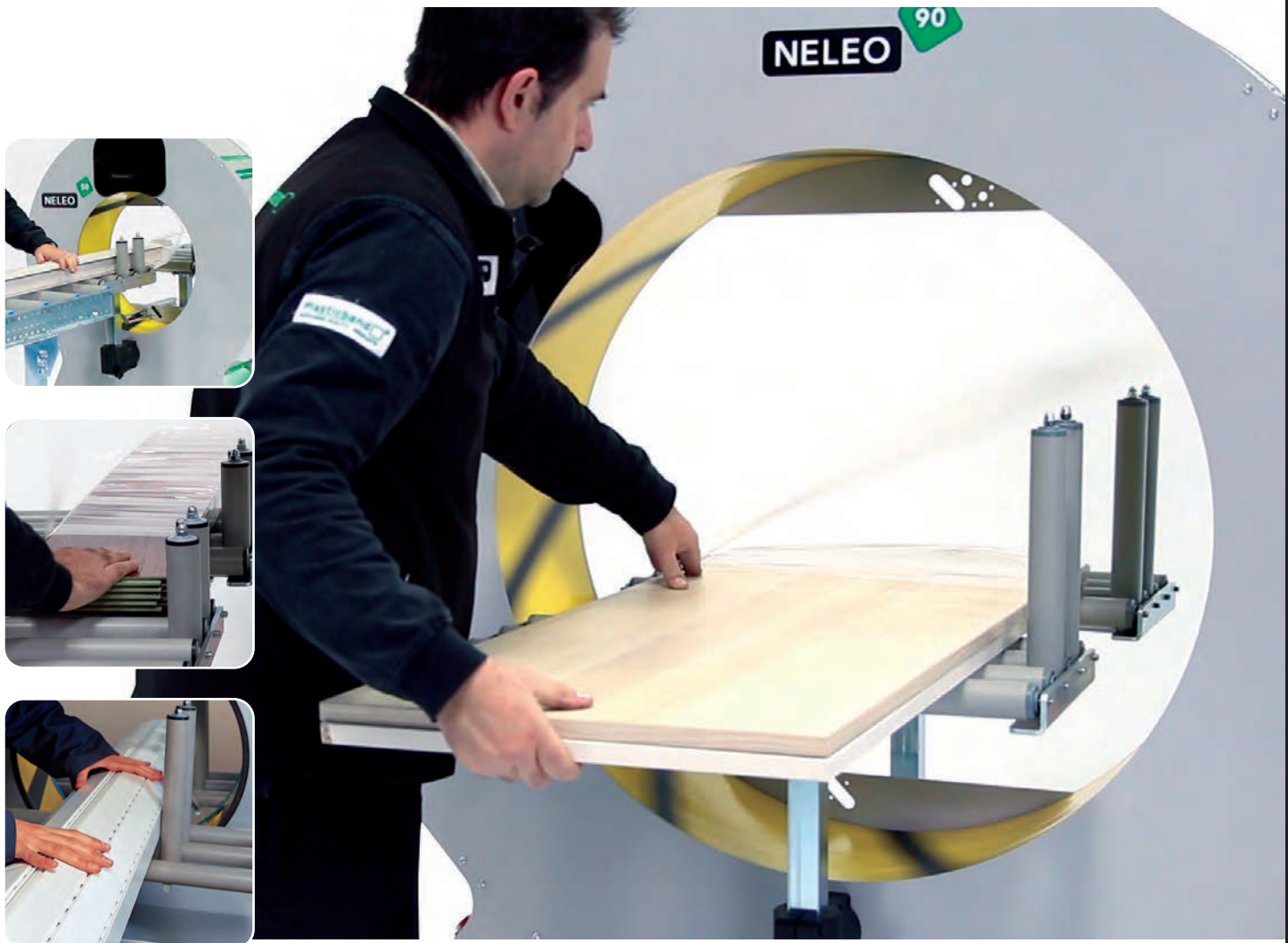
Corte y pinzado automático Automatic film cutter & clamp Coupe et pinceur automatique
